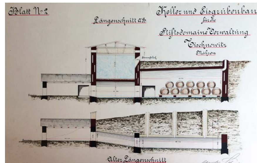
První varianta nerealizovaného projektu nového chladného hospodářství od Ferdinanda Sehnala. Řezy. Dat. 1893, sign. Ferdinand Sehnal, Stadt. – Baumeister Brünn. V první variantě připojil Sehnal k zadnímu průčelí sýpky nové příčné křídlo s lednicí a využil pro ležácký sklep barokní vinný sklep. Dole je podélný řez tímto sklepem s dlouhou šíjí ústící v dílně bednáře. (MZA v Brně)
